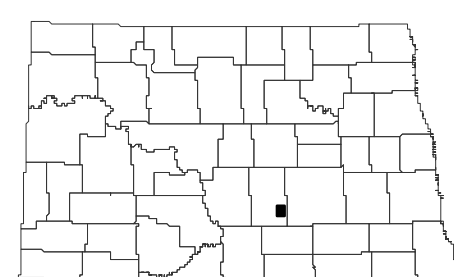
Tappen SE Quadrangle, North Dakota
