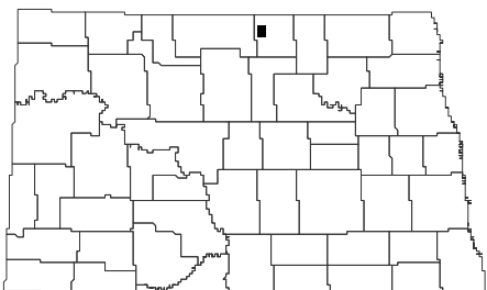
Dunseith Quadrangle, North Dakota
